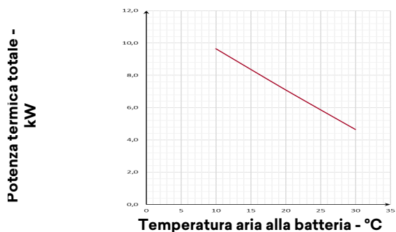
POTENZA TERMICA (3)
