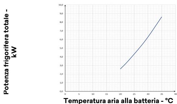
POTENZA FRIGORIFERA (4)
