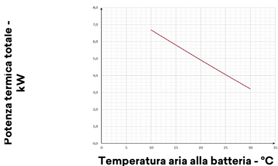
POTENZA TERMICA (3)
