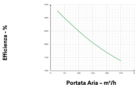
EFFICIENZA TERMICA (1)
