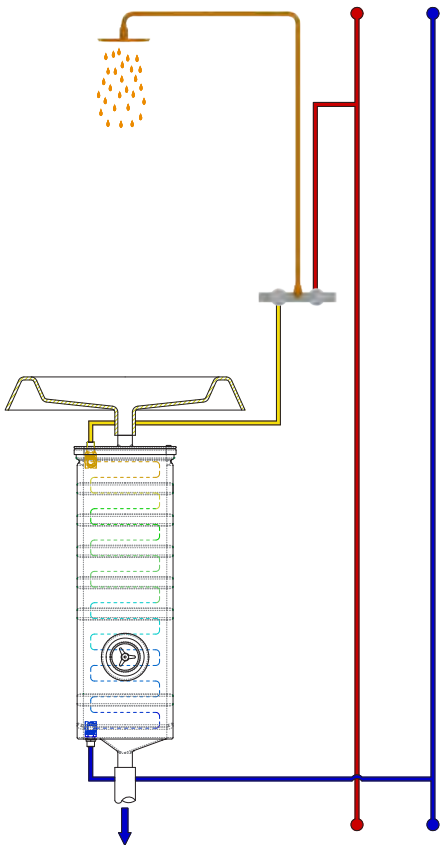
Collegamento singolo - Single connection Schema A - Diagram A
